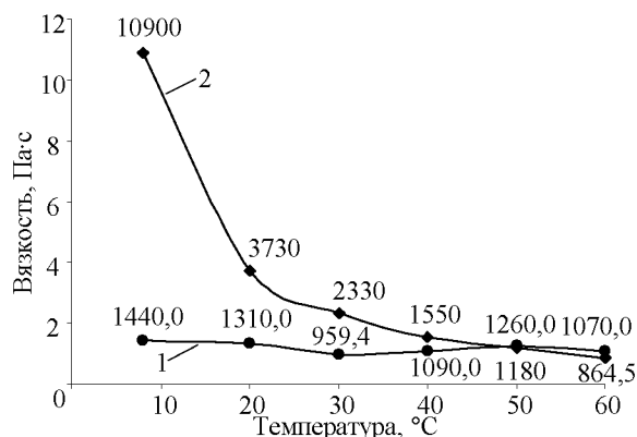
Рис.4. Зависимости упругой (1) и вязкой (2) компоненты вязкости от температуры при частоте переменной нагрузки 6 Гц (для условий неразрушенной структуры нефти)
