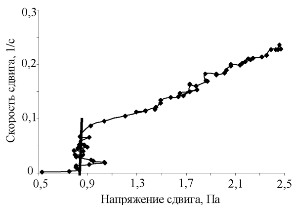
Рис.5 Зависимость скорости сдвига от напряжения сдвига при 8 °C (определение предельного напряжения сдвига \tau_0 )
