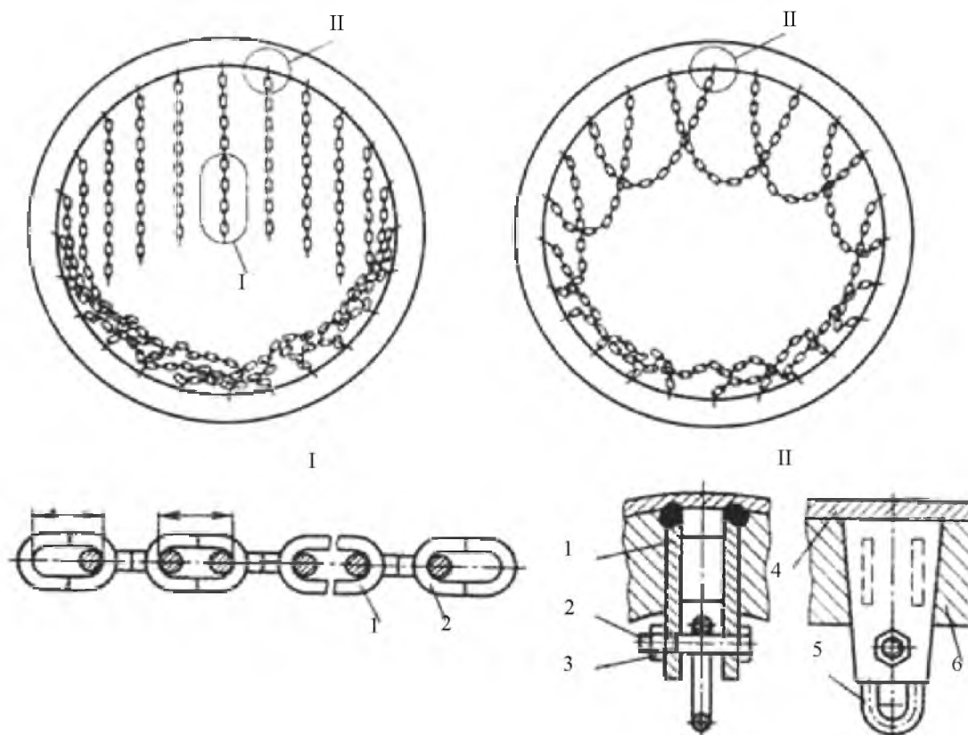
Рис.1. Цепные завесы вращающихся печей
