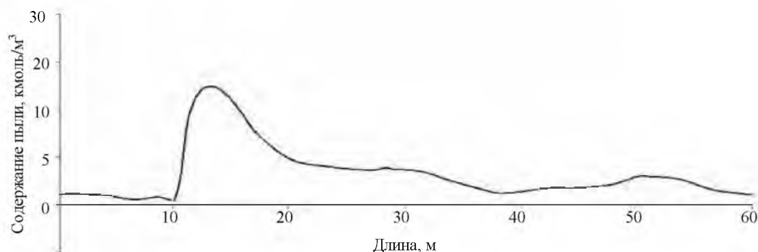
Рис.2. Изменение содержания пыли по длине печи при спекании глиноземной шихты
