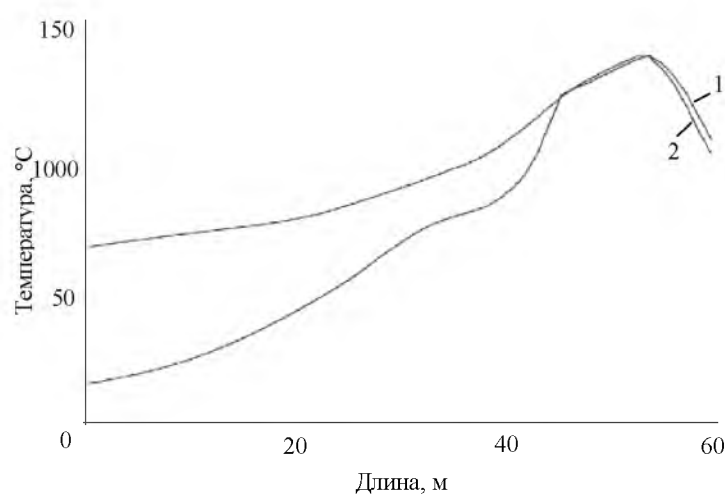
Рис.3. Температурные профили газовой (1) и твердой (2) фаз при спекании глиноземной шихты с учетом цепной завесы
