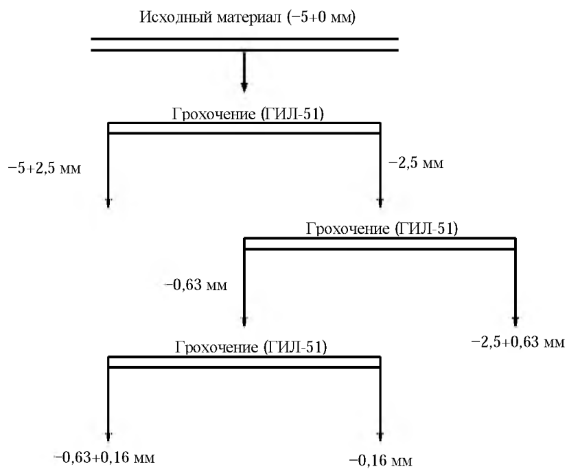
Рис. 2. Линия кондиционирования отсеков гранитного щебня
