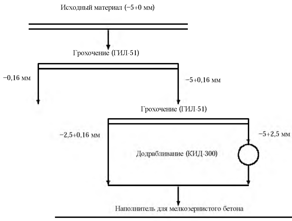
Рис.1. Линия модифицирования отсеков гранитного щебня
