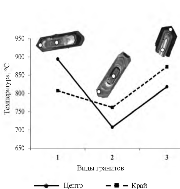
Рис.1. Эволюция температур кристаллизации циркона в гранитах Верхнеурмийского массива, рассчитанных с помощью модели «Ti-in-zircon» в центральных и краевых частях кристаллов
