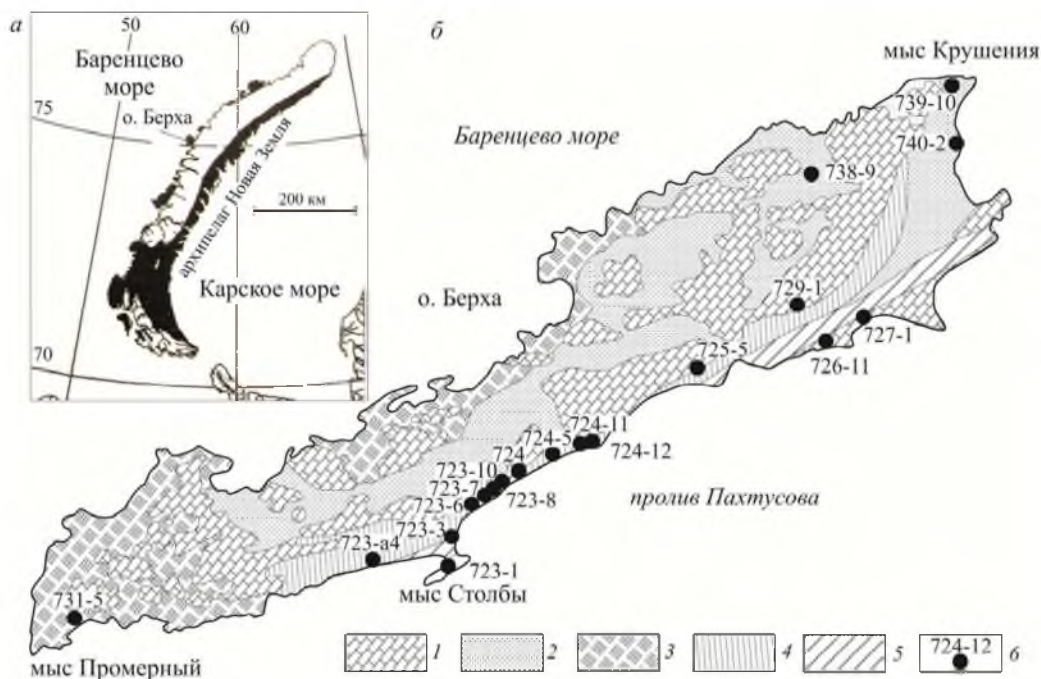
Рис.1. Местоположение острова Берха в архипелаге Новая Земля: а – карта архипелага Новая Земля; черным отмечены площади развития каменноугольно-нижнепермских отложений; б – выкопировка из геологической карты Горбовского рифового массива масштаба 1:10 000 [3] с дополнениями авторов
