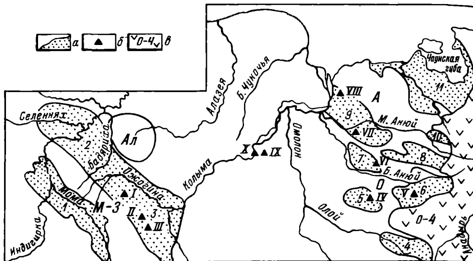
Рис. 1. Схема расположения меловых впадин а — контуры впадин; б — разрезы, изученные геологами Колымской партии ВНИГРИ; в — Охотско-Чукотский вулканогенный пояс. Структурно-фациальные области: М-3 — Момо-Зырянская (1—3); А — Алазейская; О — Олойская (4—7); А — Анойская (8—11). Структурно-фациальные зоны: 1 — Момская; 2 — Индигирская; 3 — Ожогинская; 4 — Умукевская; 5 — Ненканская; 6 — Айнахкургенская; 7 — Орловская; 8—9 — Южно-Анойская (8 — Нутесынская впадина; 9 — Камешковская впадина); 10 — Тытыльевская; 11 — Раучуанская. Разрезы: I — р. Арга—Кынрайдах; II — бассейн р. Сиялп; III — бассейн р. Зырянки; IV — р. Пеженка; V — реки Алучин, Бургахчан, Чимчемель; VI — р. Орловская; VII — р. Глубокая; VIII — р. Филиппова; IX — р. Осетровка; X — р. Мысовка у ее устья
