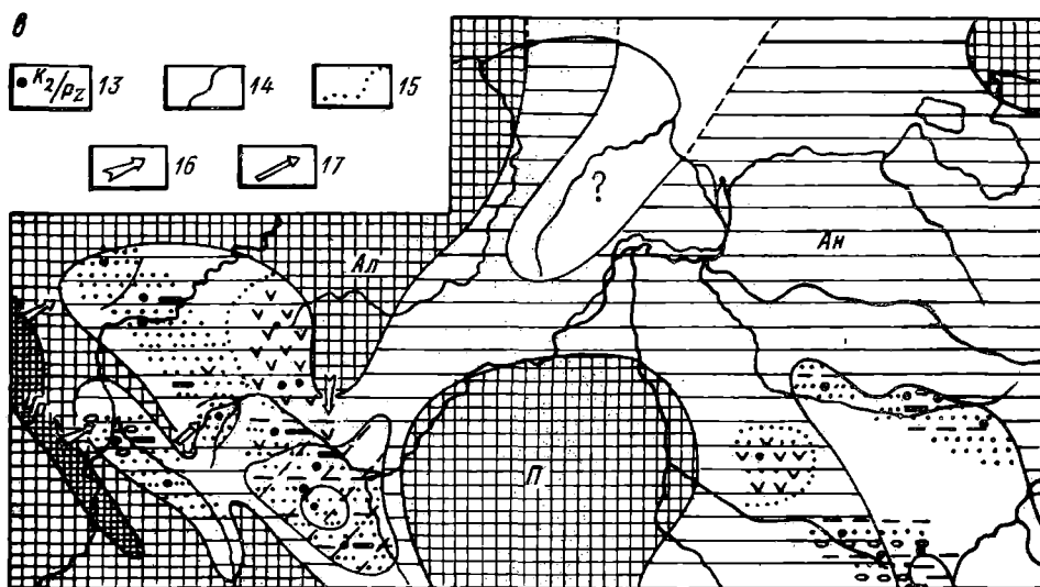
Рис. 3. Литолого-палеогеографические схемы: а — берриасского и валанжинского веков; б — готеривского и барремского веков; в — аптского века
